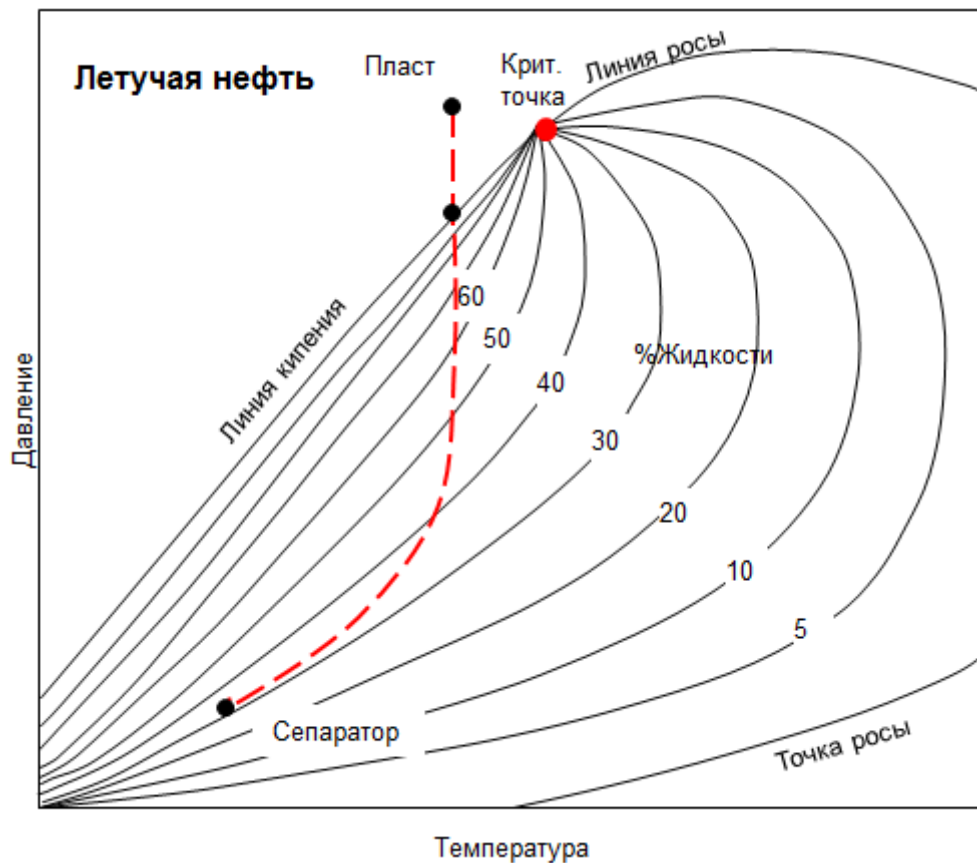
Рисунок 2. График изолиний, характеризующих модель «летучей» нефти
