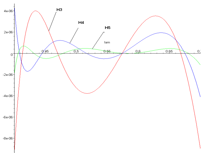
Рисунок 1. Графики функций H_3 , H_4 и H_5 для стекла N-BK7
