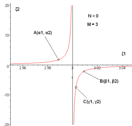
Рисунок 4б. Точки A , B и C лежат на равнобочной гиперболе, N < 0
