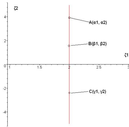
Рисунок 3. Точки A , B и C лежат на вертикальной прямой: \alpha_1 = \beta_1 = \gamma_1
