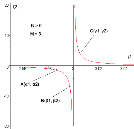
Рисунок 4а. Точки A , B и C лежат на равнобочной гиперболе, N > 0
