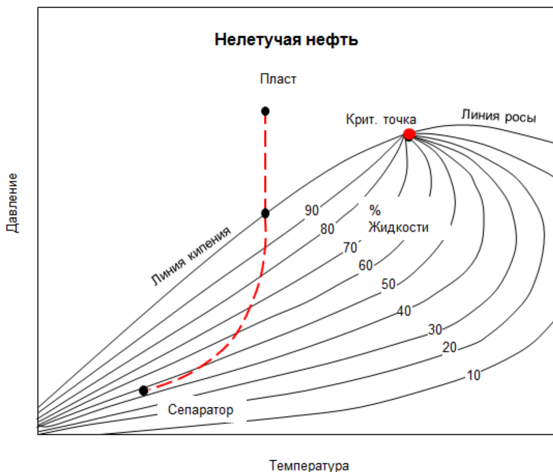
Рисунок 1. График изолиний, характеризующих модель «black oil»
