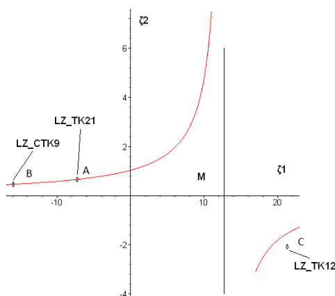
Рисунок 6. График взаимного расположения стекол
