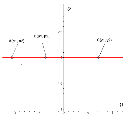
Рисунок 2. Точки А, В и С лежат на горизонтальной прямой: \alpha_2 = \beta_2 = \gamma_2
